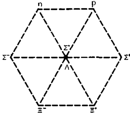
the baryon octet
